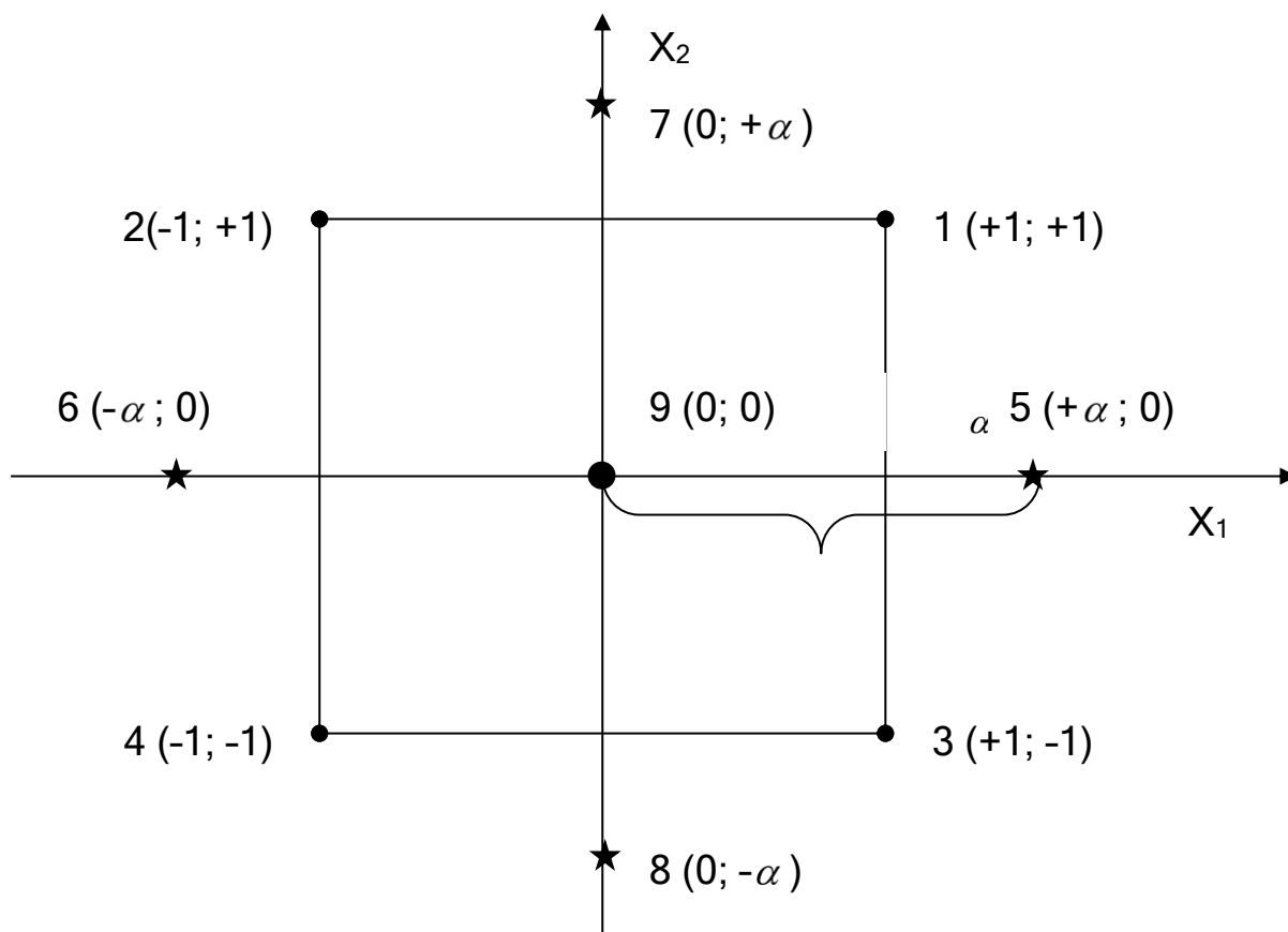
Рис. 1. Схема центрального композиционного плана второго порядка для двух факторов
