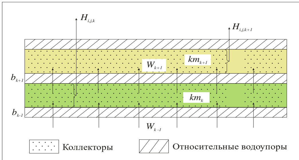
Рис. 6. Расчетная схема
