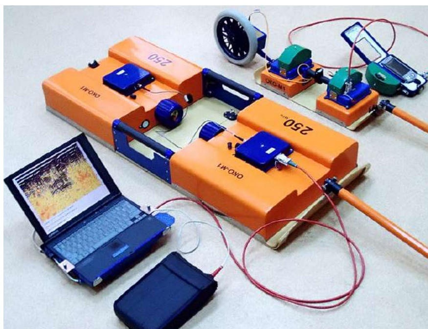
Рисунок 2.7 – Георадар «ОКО-2»
