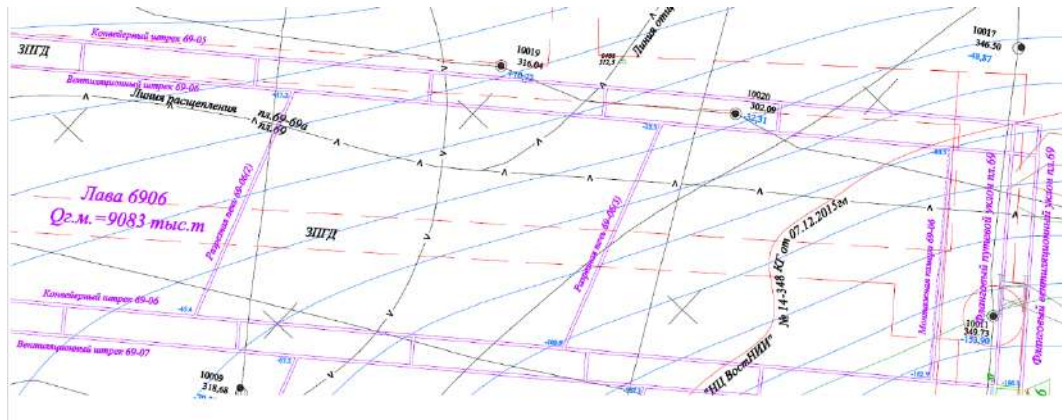
Рисунок 4.6 - Выкопировка из плана горных работ (участок конвейерного штрека 69-05 в зоне ПГД)
