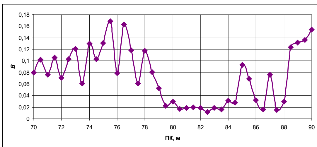
Рисунок 2.9 – График распределения коэффициента амплитуд B ЕЭМИ на участке 1 (Путевой ствол) по компоненте X
