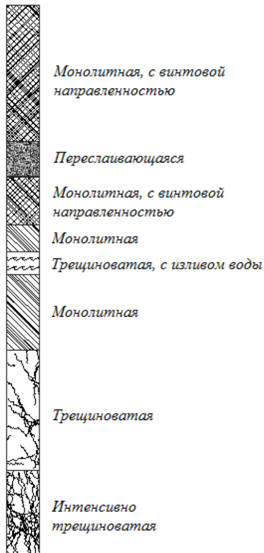
Рисунок 2.3 – Иерархическая организация породного массива
