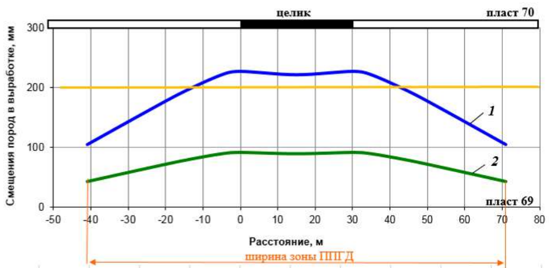
Рисунок 4.7 – Смещения кровли конвейерного штрека 69-05, закрепленного анкерной крепью и расположенного по пласту 69 в зоне ПГД от целика по пласту 70: 1 – в зоне влияния лавы 69-05; 2 – до начала отработки запасов выемочного столба 69-06
