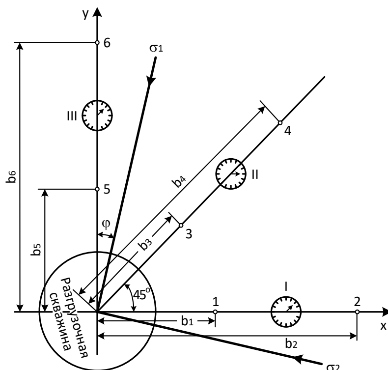
Рисунок 2.18 – Схема установки приборов и частичной разгрузки массива горных пород: 1-6 – реперы; I-III – индикаторы часового типа; b_1 - b_6 – расстояния от оси скважины до репера; \varphi – угол между вертикальной осью координат и направлением вектора максимального напряжения
