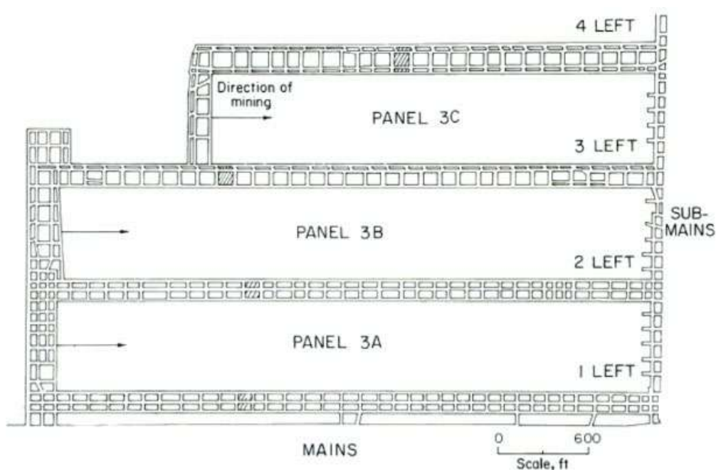
Рисунок 1.10 – Переход подготовки выемочных участков от трех к четырем штрекам
