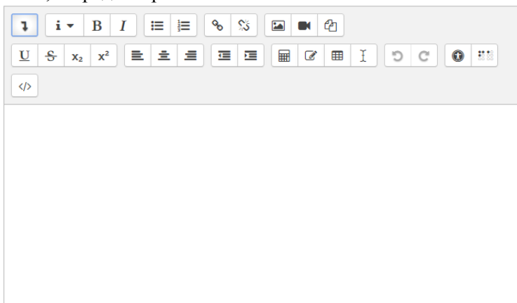
Рис. 3. Текстовый редактор
