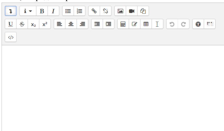
Рис. 3. Текстовый редактор
