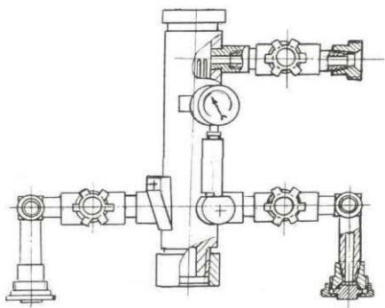
Рисунок 5.8 - Головка цементировочная
