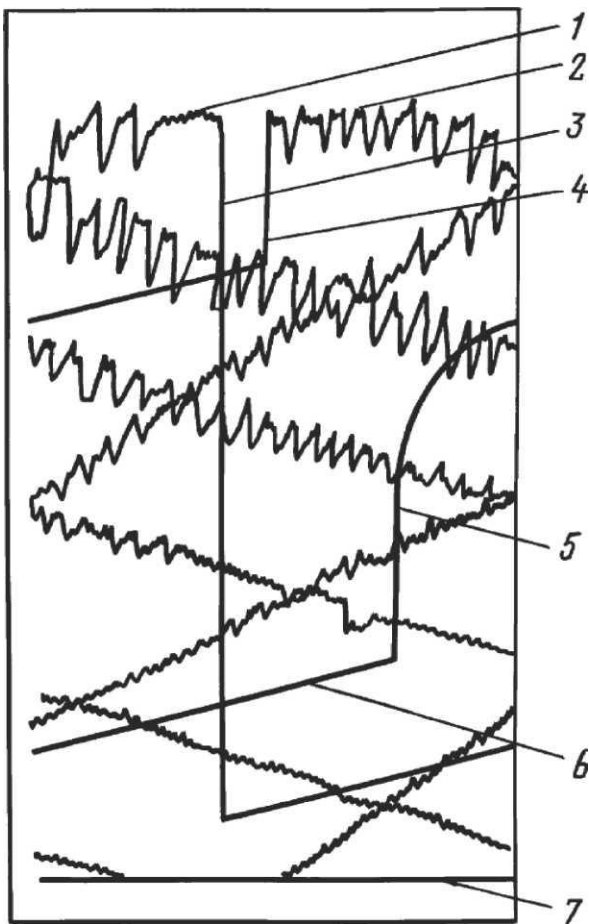
Рисунок 7.8 -Пример диаграммы, записанной с помощью глубинного манометра поршневого типа МП-3М при испытании пласта: 1, 2 - гидростатическое давление в скважине соответственно до испытания и после него; 3 - открытие приемного клапана; 4 - открытие уравнительного клапана; 5 - кривая восстановления забойного давления; 6 - приток; 7 - начало отсчета давления (нулевая линия).
