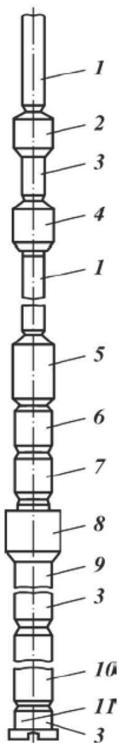
Рисунок 7.3 - Схема пластоиспытателя, спускаемого на бурильных трубах: 1 - бурильные трубы; 2 - циркуляционный клапан; 3 - глубинные манометры; 4 - запорный поворотный клапан; 5 - гидравлический испытатель пластов; 6 - ясс; 7 - безопасный переводник; 8 - пакер; 9 - фильтр; 10 - хвостовик; 11 - опорный башмак (пята).
