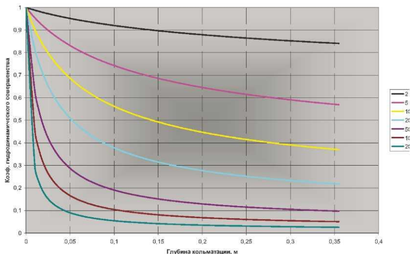
Рисунок 2.5 - Влияние параметров зоны кольтации на коэффициент гидродинамического совершенства скважины при p_2 = 1 . p_1 - степень снижения проницаемости (2, 5, 10, 20, 50, 100, 200).
