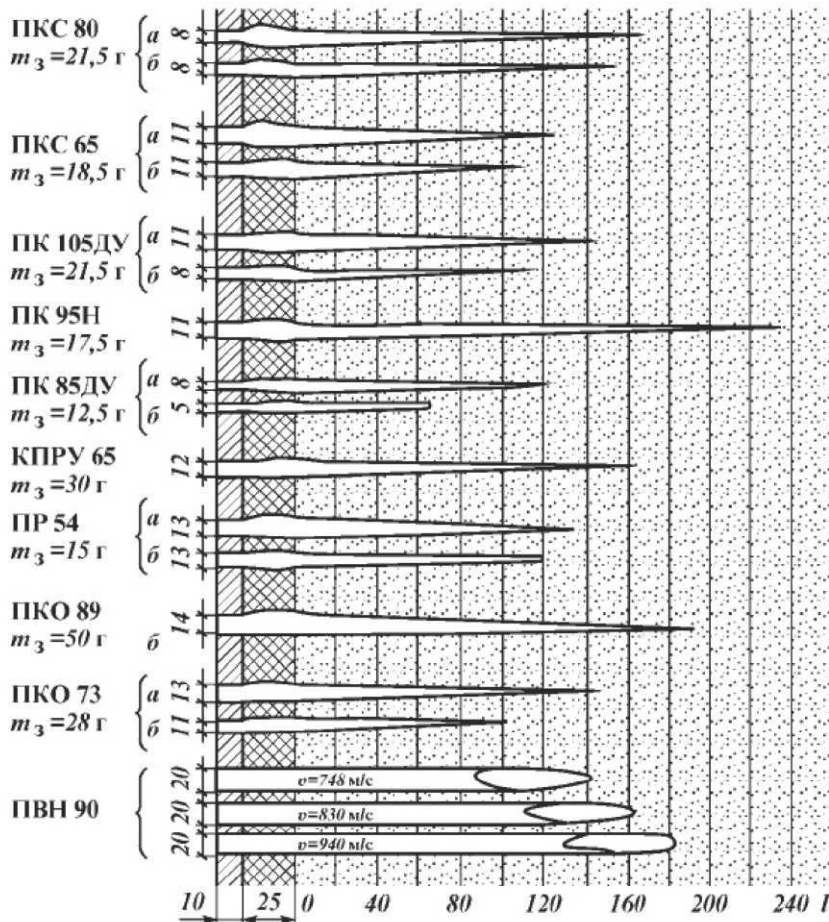
Рисунок 6.1 - Размеры перфорационных каналов при давлении атмосферном (а) и 30 МПа (б).
