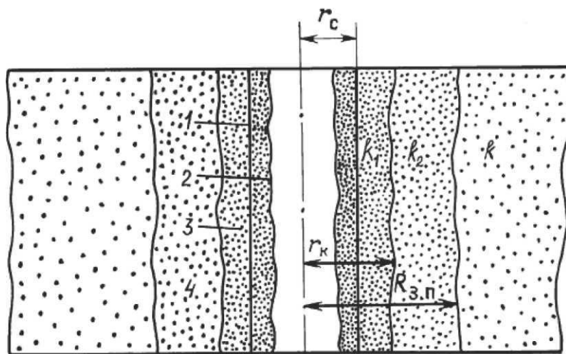
Рисунок 2.4 - Схемы прискважинной зоны пласта после вскрытия его бурением:
