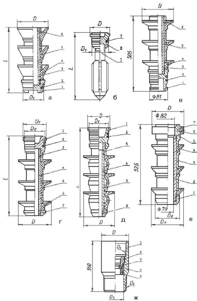
Рисунок 5.14 - Разновидности ПДМ: а - пробка ПДМ.050; б-пробка ПДМ.060; в- пробка ПДМ.070; г- пробка дополнительная ПДМ.070-01; д- пробка дополнительная ПДМ.070-02;е- пробка проточная ПДМ.090-01; ж- патрубок ПДМ.080
