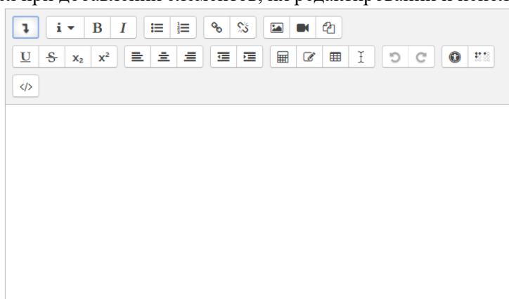
Рис. 3. Текстовый редактор
