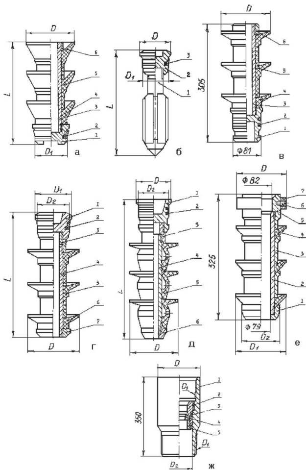
Рисунок 5.14 - Разновидности ПДМ: а - пробка ПДМ.050; б-пробка ПДМ.060; в- пробка ПДМ.070; г- пробка дополнительная ПДМ.070-01; д- пробка дополнительная ПДМ.070-02;е- пробка проточная ПДМ.090-01; ж- патрубок ПДМ.080
