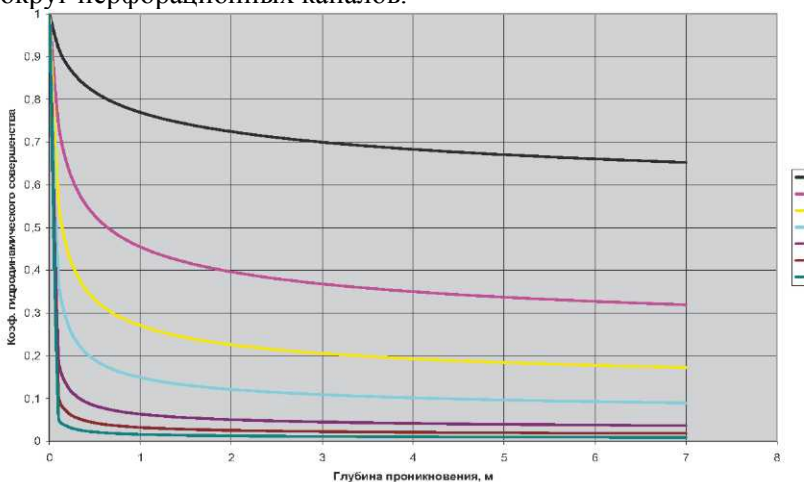
Рисунок 2.6 - Влияние параметров зоны проникновения фильтра на коэффициент гидродинамического совершенства скважины при p_1 = 1 . p_2 - степень снижения проницаемости (2, 5, 10, 20, 50, 100, 200)
