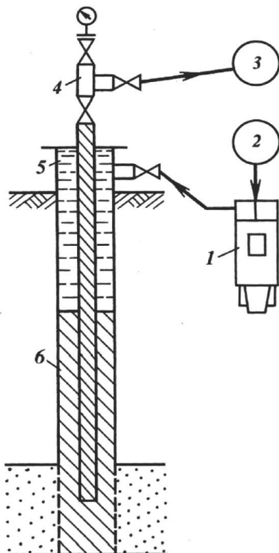
Рисунок 8.1 - Схема обвязки оборудования для замены бурового раствора водой: 1 - насосный агрегат; 2 - емкость для воды (или водовод); 3 - емкость для сбора бурового раствора; 4 - устье скважины; 5 - вода; 6 - буровой раствор.
