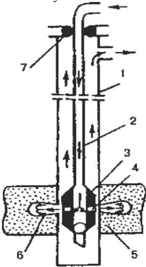
Рисунок 6.2 - Схема перфорации в скважине гидropескоструйным методом: 1-обсадная колонна; 2-НКТ; 3-АП; 4-насадка; 5-пласт; 6-каналы ГПП; 7-сальник.
