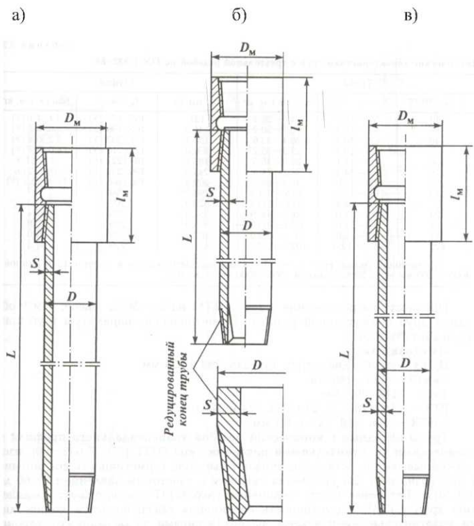
Рисунок 4.1. Трубы обсадные муфтовые
