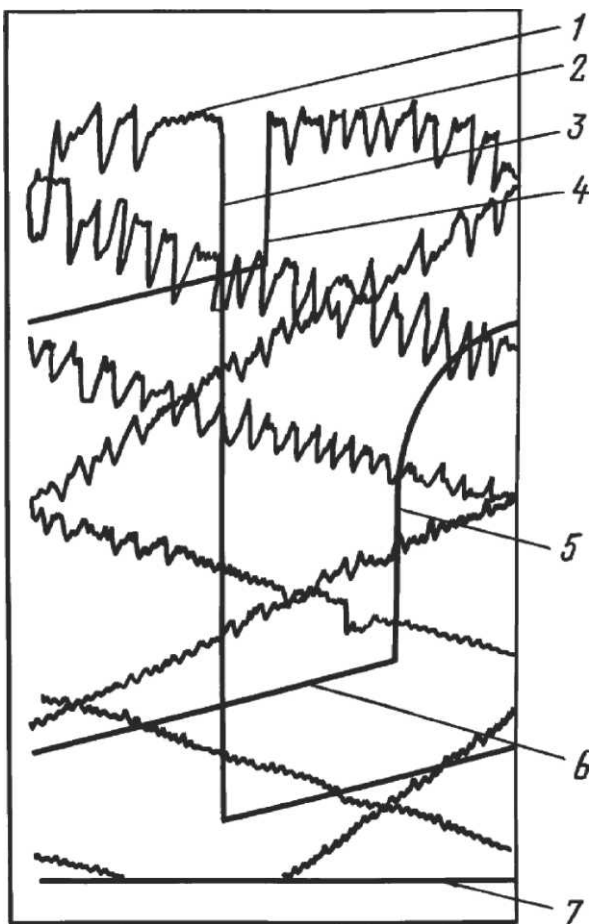
Рисунок 7.8 -Пример диаграммы, записанной с помощью глубинного манометра поршневого типа МГП-3М при испытании пласта: 1, 2 - гидростатическое давление в скважине соответственно до испытания и после него; 3 -открытие приемного клапана; 4 - открытие уравнительного клапана; 5 - кривая восстановления забойного давления; 6 - приток; 7 - начало отсчета давления (нулевая линия).
