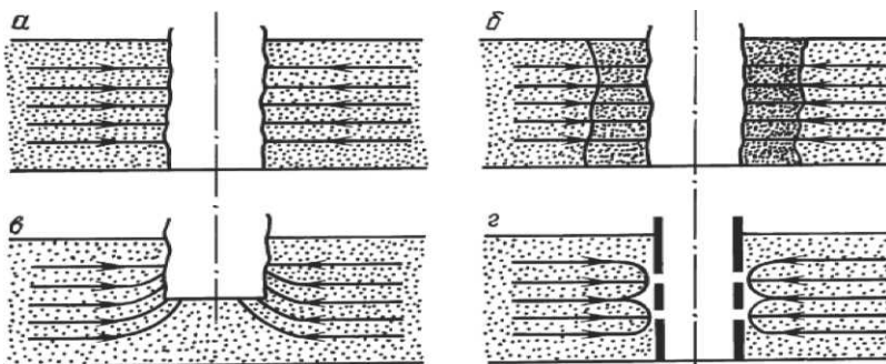
Рисунок 2.3 - Схемы притока в гидродинамически совершенную (а) и гидродинамически несовершенные скважины по качеству (б), степени (в) и характеру (г) вскрытия продуктивного горизонта.
