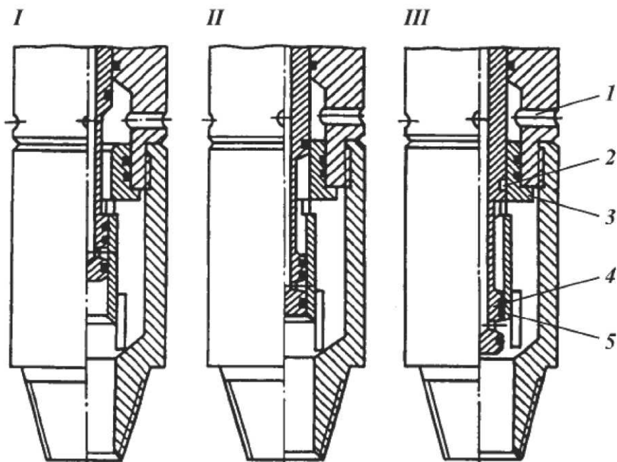
Рисунок 7.5 - Этапы работы клапанов ИПГ: 1 - уравнильные каналы; 2 - уплотнитель уравнильного клапана; 3, 5 - гильзы соответственно уравнильного и приемного клапанов; 4 - приемный клапан.
