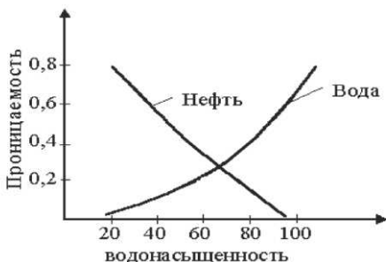
Рисунок 1.2 Изменение относительной проницаемости образца в зависимости от его водонасыщенности
