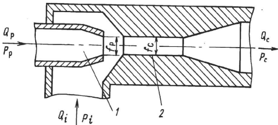
Рисунок 8.4 - Схема струйного аппарата: 1 - рабочая насадка; 2 - приемная камера с диффузором.
