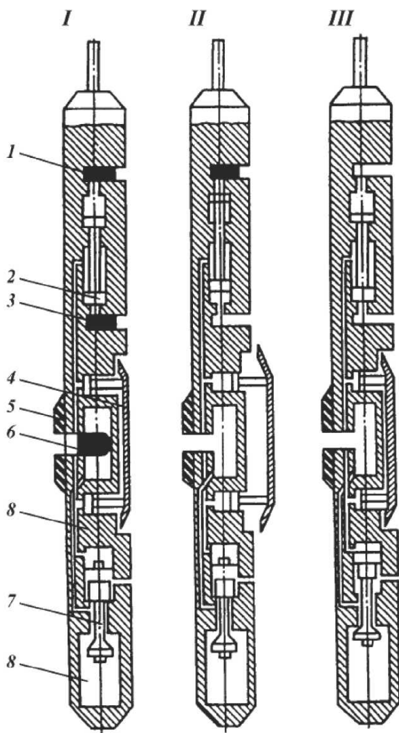
Рисунок 7.2 - Этапы работы опробователя на кабеле:
