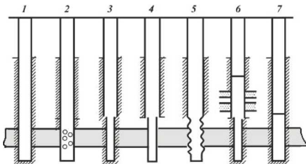
Рисунок 3.2 - Типы конструкций эксплуатационных колонн: 1, 2 - сплошные колонны, зацементированные соответственно через башмак и специальные отверстия над пластом; 3, 4 - зацементированные колонны с хвостовиком; 5 - колонна спущенная до пласта (эксплуатация с открытым забоем); 6, 7 - комбинированные колонны спущенные секциями
