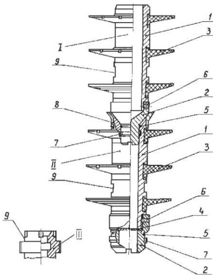
Рисунок 5.15 - Комплект разделительных пробок с фиксатором КРПФ 140-146: I-пробка верхняя ПРВФ; II-пробка нижняя ПРНФ; III- кольцо-стоп; 1-корпус; 2-наконечник; 3-манжета; 4-диафрагма; 5-уплотнительное кольцо; 6-штифт; 7- кольцо разрезное (фиксатор); 8- воронка; 9- место маркировки.
