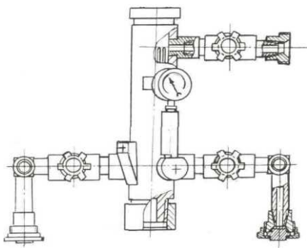
Рисунок 5.8 - Головка цементировочная
