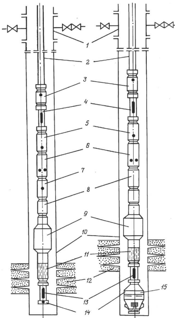
Рисунок 7.4 - Схема пакерования при работе с КИИ: 1 - колонная головка; 2 - НКТ; 3 - циркуляционный клапан; 4 - верхний манометр; 5 -запорно-поворотный клапан; 6 - испытатель пластов; 7 - ясс; 8 - пробоотборник; 9 - пакер; 10 - обсадная колона; 11 - фильтр; 12 - пласт; 13 - манометр; 14 - опорная плита; 15 - башмак.
