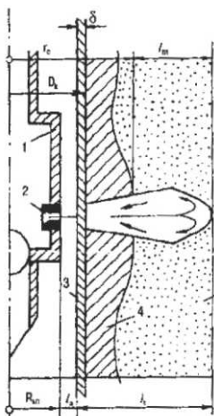
Рисунок 6.4 - Схема формирования канала ГПП в скважине: 1 - гидropескоструйный аппарат; 2 - насадка; 3 - колонна; 4 - цементное кольцо; 5 - пласт.
