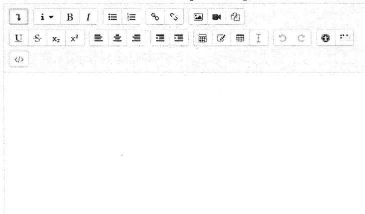
Рис. 3. Текстовый редактор
