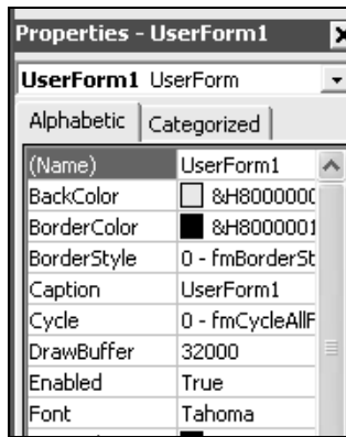
Рис. 1.3. Окно свойств
