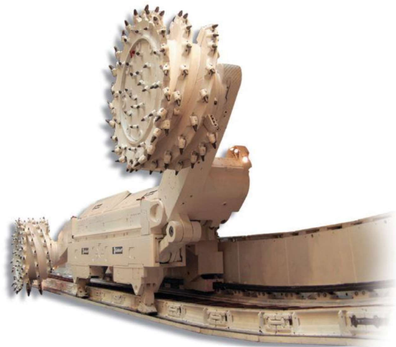
Werksfoto eines Walzenschrämladers (Bildspende der Firma Gebr. Eickhoff Maschinenfabrik und Eisengießerei, Bochum)
