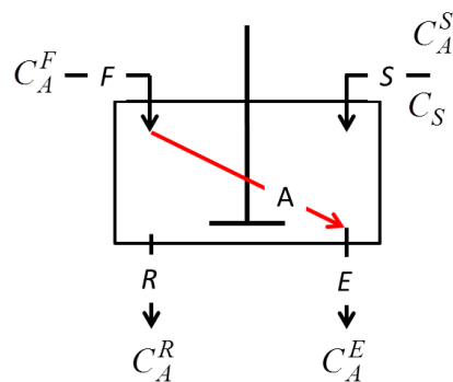
Рис. 2. Схема экстракции
