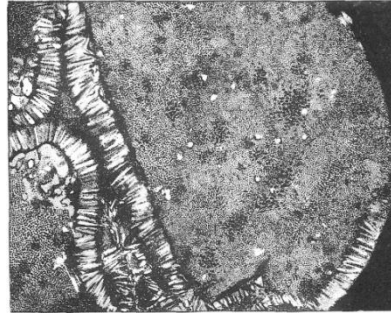
Крустификационный цемент
