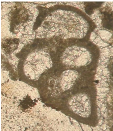
Раковина фораминиферы
