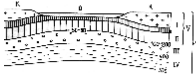
Рис. 3.4. Схема соотношения литосферы, астеносферы и тектоносферы.
