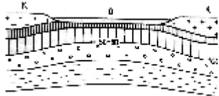
Рис. 3.4. Схема соотношения литосферы, астеносферы и тектоносферы.
