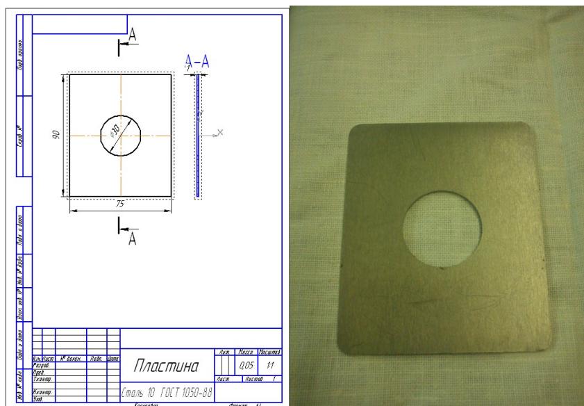
Рис.2. Образец-пластина (круг): а)чертеж б)общий вид
