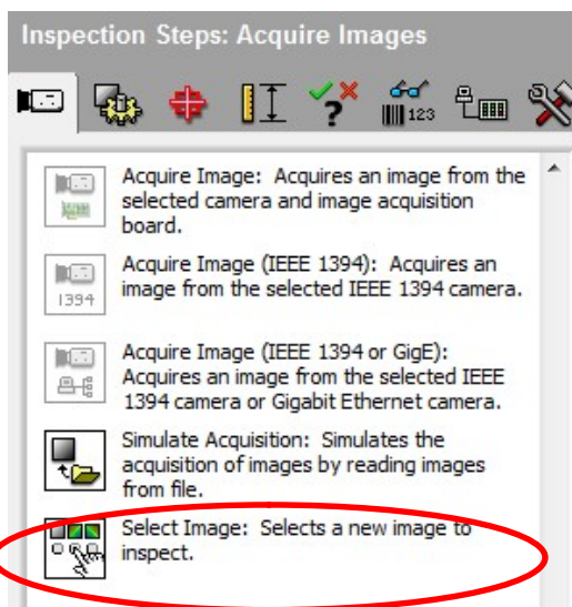
Рис.5 Функция выбора изображения
