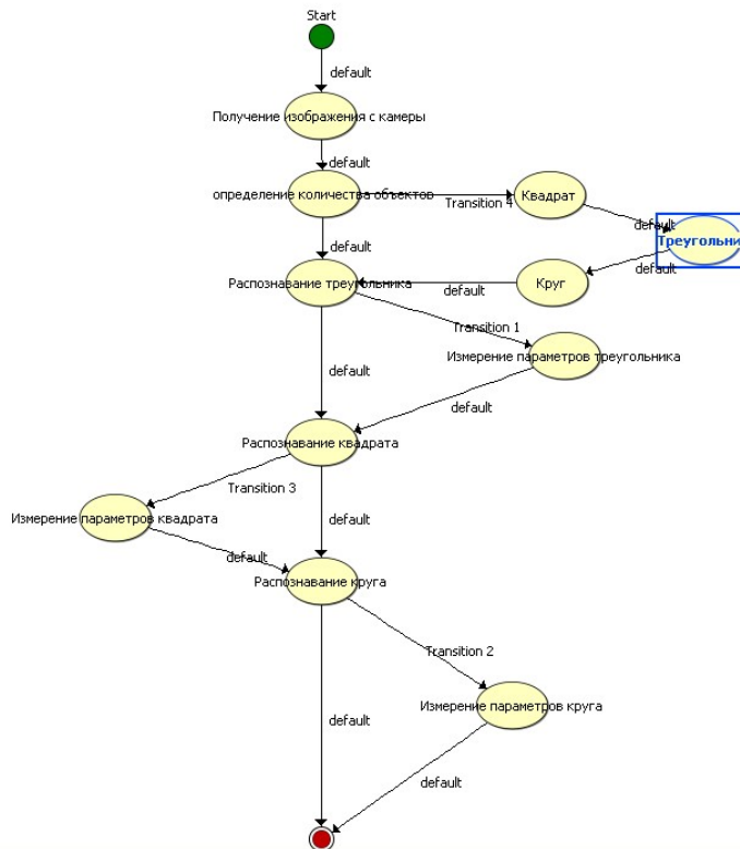
Рис.1 Алгоритм управляющей программы
