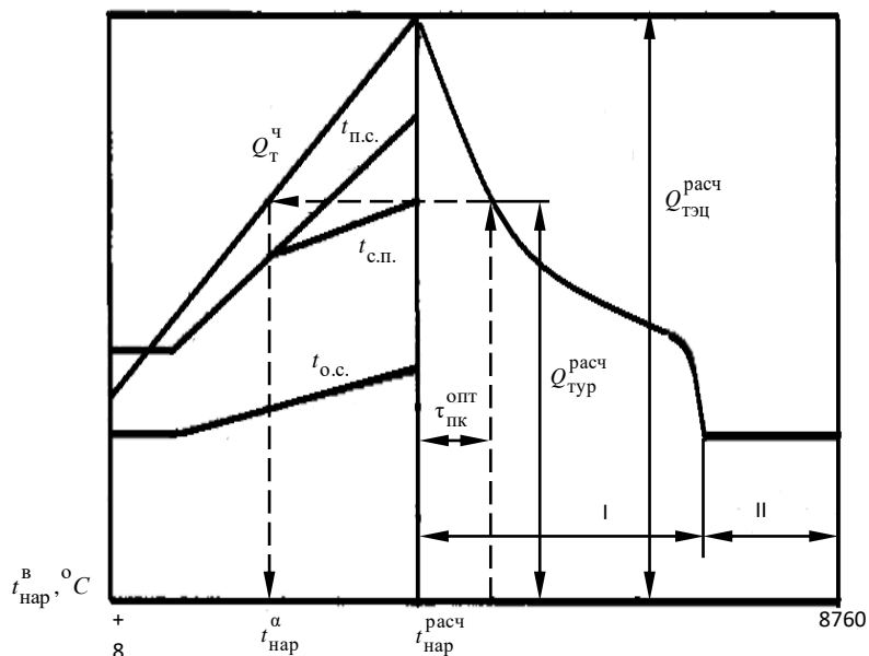
Рис. 6. Годовой график отпуска тепла по продолжительности:
