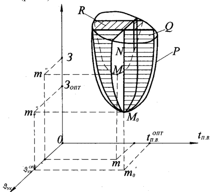
Рис 2. Геометрическая интерпретация отдельного и совместного определения оптимальных значений t_{пв} и \vartheta_{yx} .
