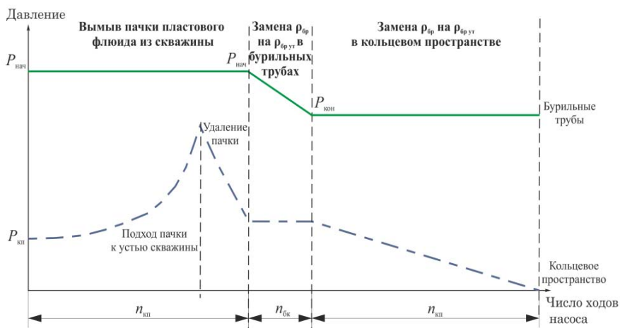
Рис. 1. График изменения давления в буровых трубах и кольцевом пространстве при использовании метода «бурильщика»
