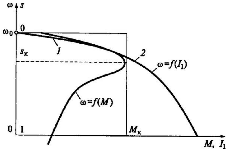
Рис.2. Механическая и электромеханическая характеристики спроектированного двигателя
