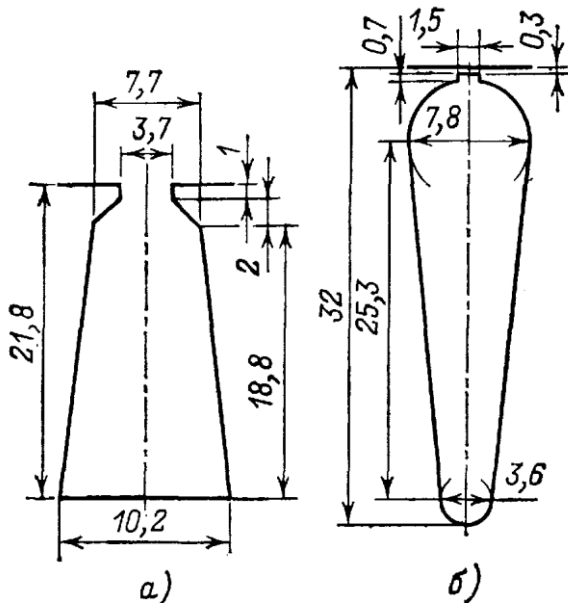
Рис.1. Пазы спроектированного двигателя: а – статора; б – ротора
