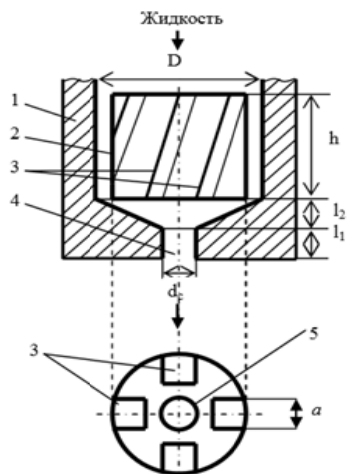
Рис. 4.2. Центробежно-струйная форсунка: 1 – корпус; 2 – вкладыш; 3 – каналы завихряющие; 4 – сопло; 5 – центральный канал
