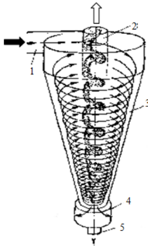
Рис. 1.1. Циклон:
