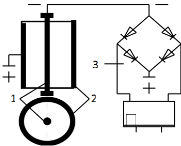
Рис. 3.1. Схема трубчатого электрофильтра
