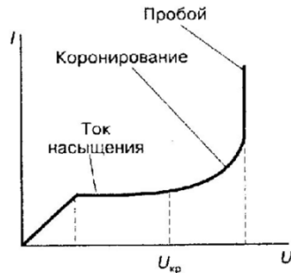
Рис. 3.2. Вольтамперная характеристика электрофильтра
