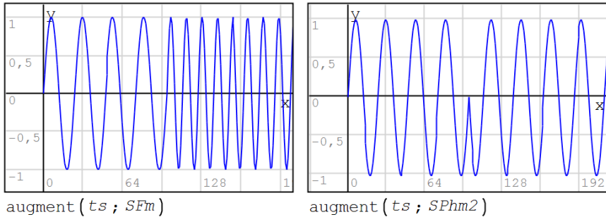
Рис. 18. Радиоимпульсы с частотной и фазовой модуляцией
