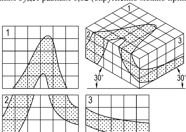
Рис. 8. Построение блок-диаграммы в прямоугольной изометрической аксонометрической проекции
