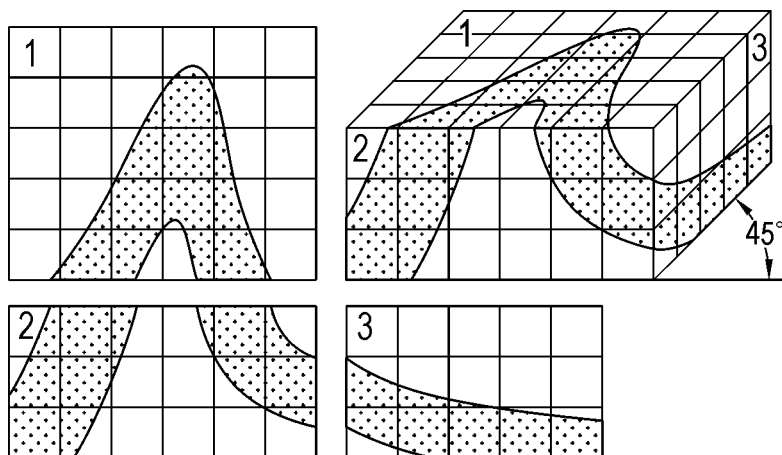
Рис. 7. Построение блок-диаграммы в косоугольной аксонометрической проекции
