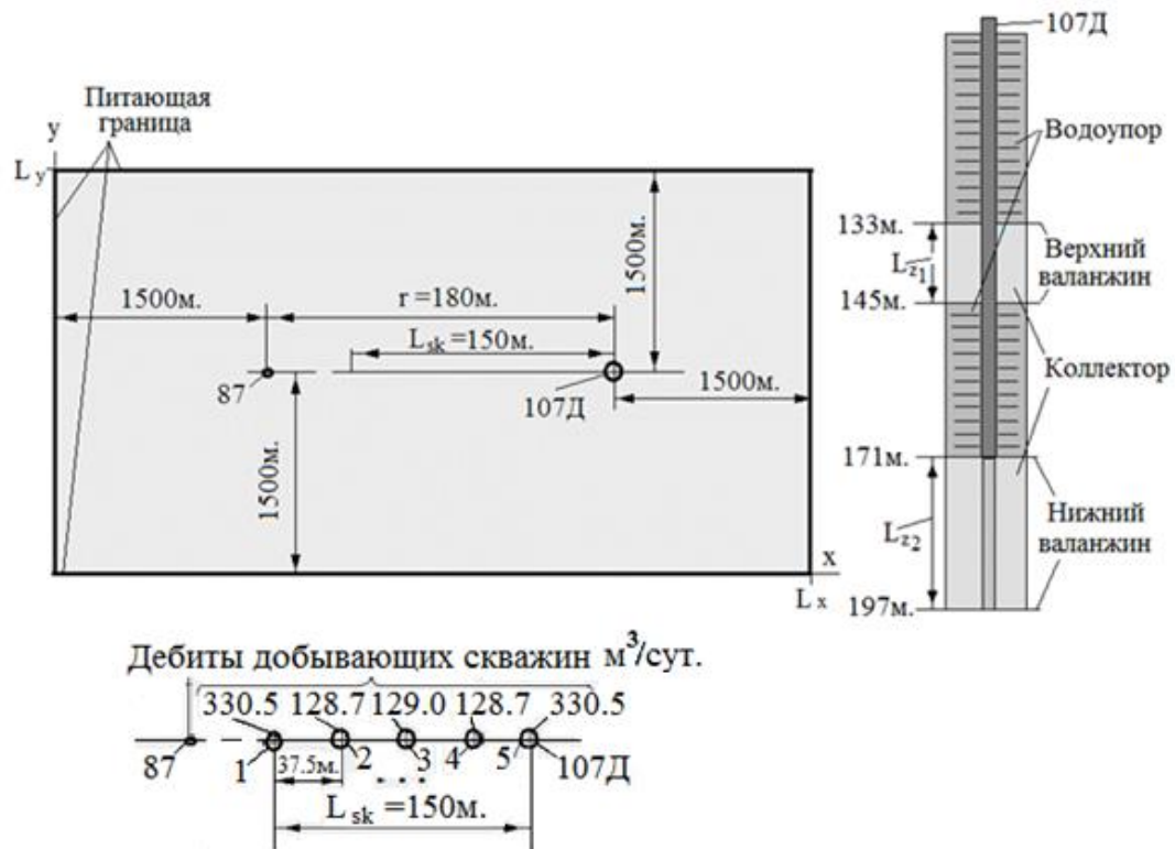
Рисунок 4.2 — Схема расположения оптимального числа добывающих скважин и полученные дебиты [46]
