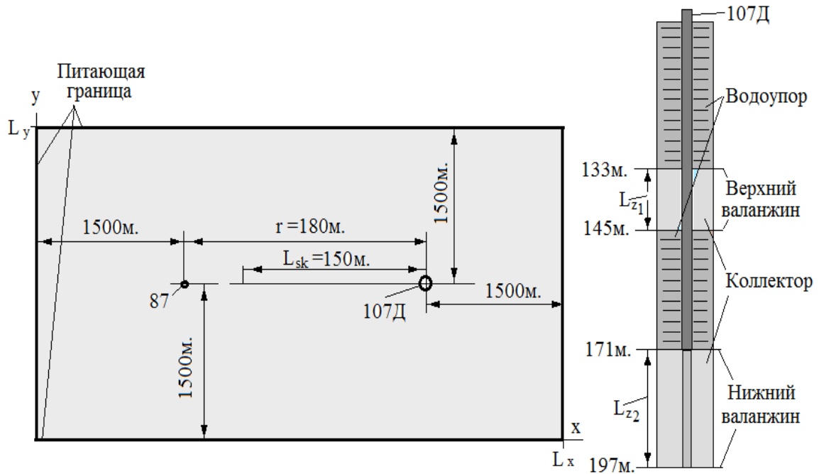
Рисунок 2.6 — Схема месторождения (составлено автором)
