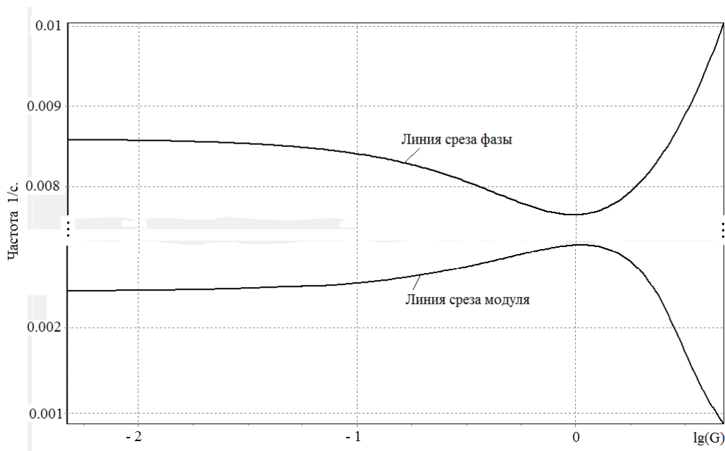
Рисунок 3.21 — Анализ устойчивости замкнутой системы (составлено автором)
