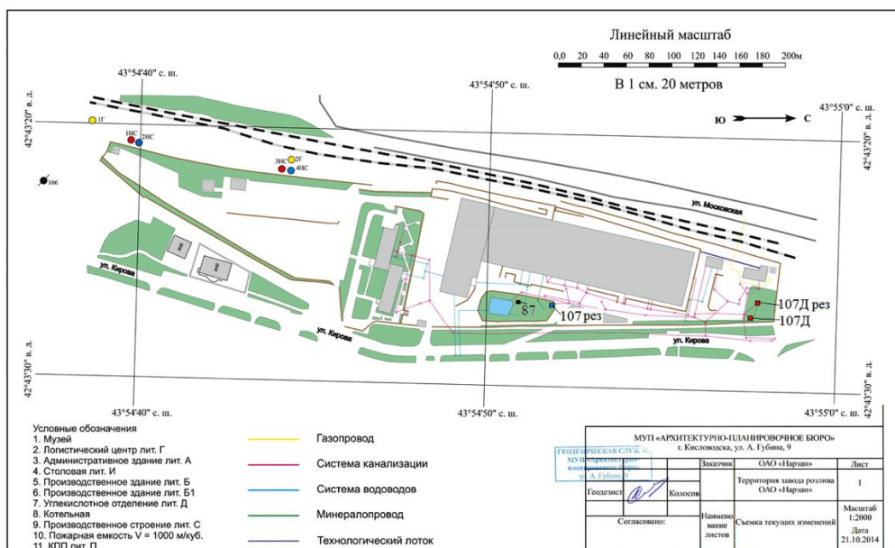
Рисунок 1.6 — Схема скважин [17]
