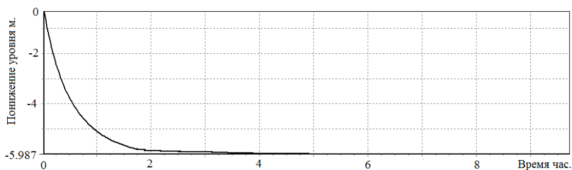
Рисунок 3.2 — График изменения уровня в зоне расположения третьей добывающей скважины (составлено автором)
