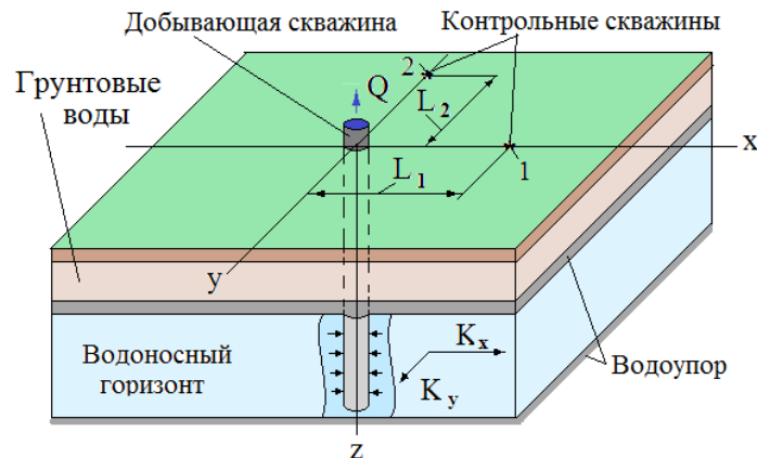
Рисунок 2.2 — Расположение добывающей и контрольной скважин [41]
